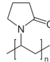
Polyvinylpyrrolidon (PVP)
