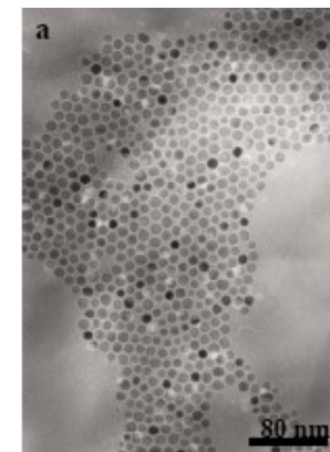
Cu nanoparticles
