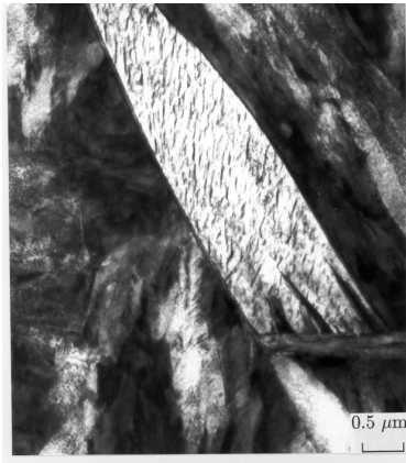
Unterer Bainit mit Karbidausscheidungen in „sub-unit“ mit bevorzugter Orientierung
