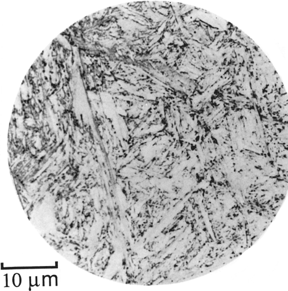
Martensit
